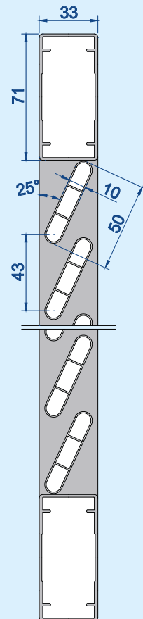
Vertikalschnitt: Maßstab 1:3
