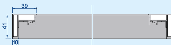
Horizontalschnitt: Maßstab 1:3
